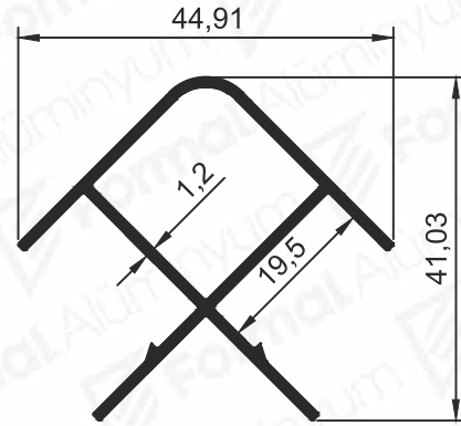
Pr.No: 8801 0,447 kg/m
