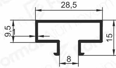
Pr.No: 8575 0,205 kg/m
