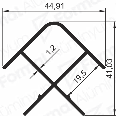
Pr.No: 8801 0,447 kg/m
