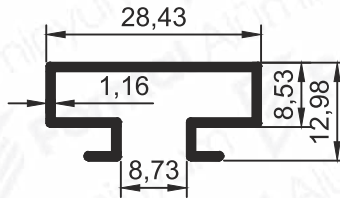
Pr.No: 8148 0,240 kg/m
