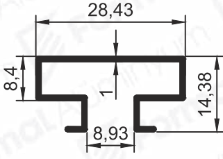
Pr.No: 1036 0,213 kg/m
