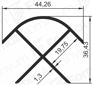
Pr.No: 8596 0,472 kg/m
