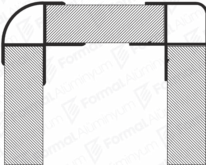
Pr.No: 8596
