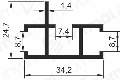
Pr.No: 8158 0,382 kg/m
