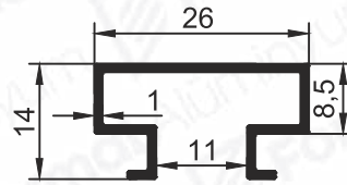
Pr.No: 8791 0,189 kg/m
