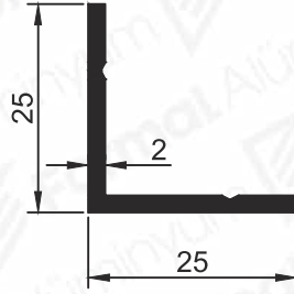
Pr.No: 1224 0,257 kg/m
