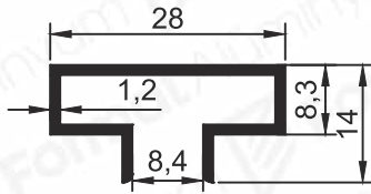
Pr.No: 8151 0,229 kg/m
