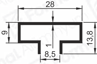
Pr.No: 2158 0,193 kg/m
