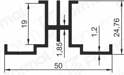
Pr.No: 1621 0,445 kg/m
